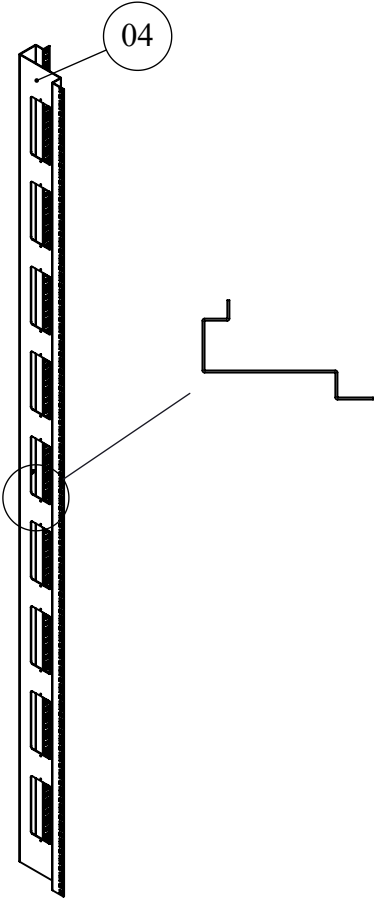
THANH LẮP THIẾT BỊ
