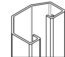
XTRUK 9 SIDES MAX LOAD 1350kg
