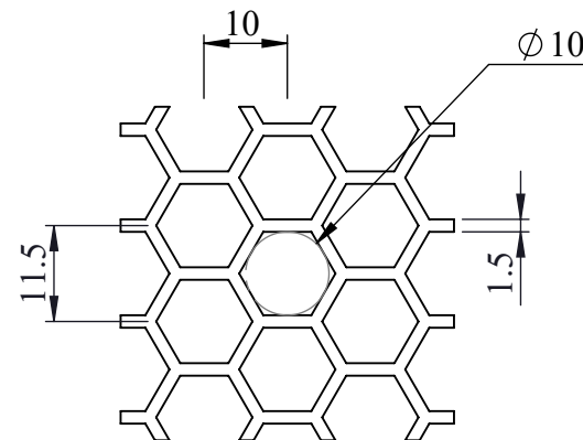
DETAIL A: LƯỚI LỖ ĐỘT LỤC GIÁC >80% THÔNG THOÁNG KHÍ
